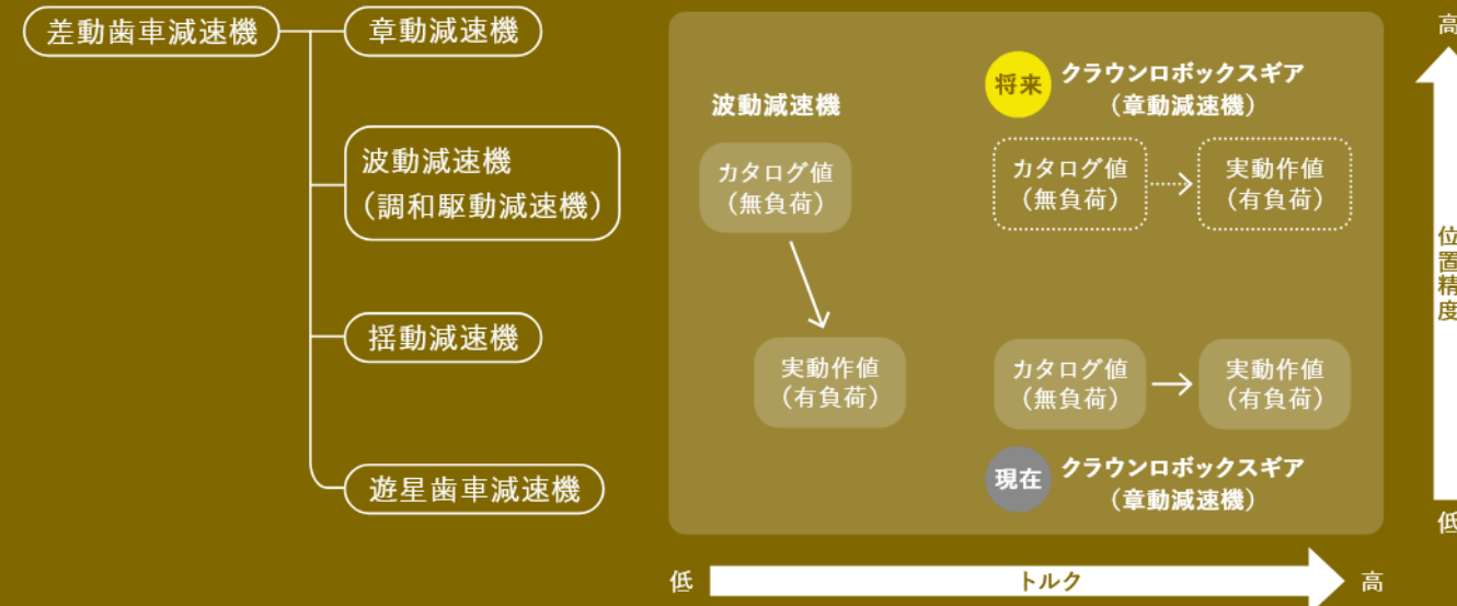
小型減速機における負荷(実動作)時の各減速機のポジション
